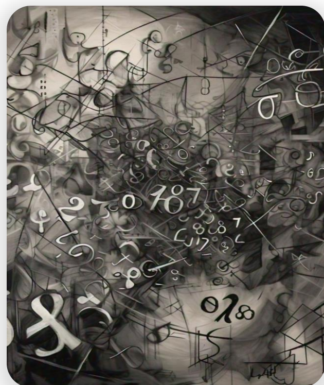
Algoritmos
